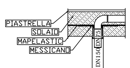
RIPRISTINO DEGLI ATTRAVERSAMENTI DEL SOLAIO - RIMOZIONE DELLO SCARICO ESISTENTE - POSA DI MESSICANO - COPERTURA CON GUAINA IMPERMEABILIZZANTE MAPELASTIC - INSTALLAZIONE DI NUOVA TUBAZIONE DI SCARICO
