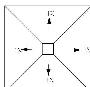
POSA DI PILETTA A PAVIMENTO CON PENDENZA
