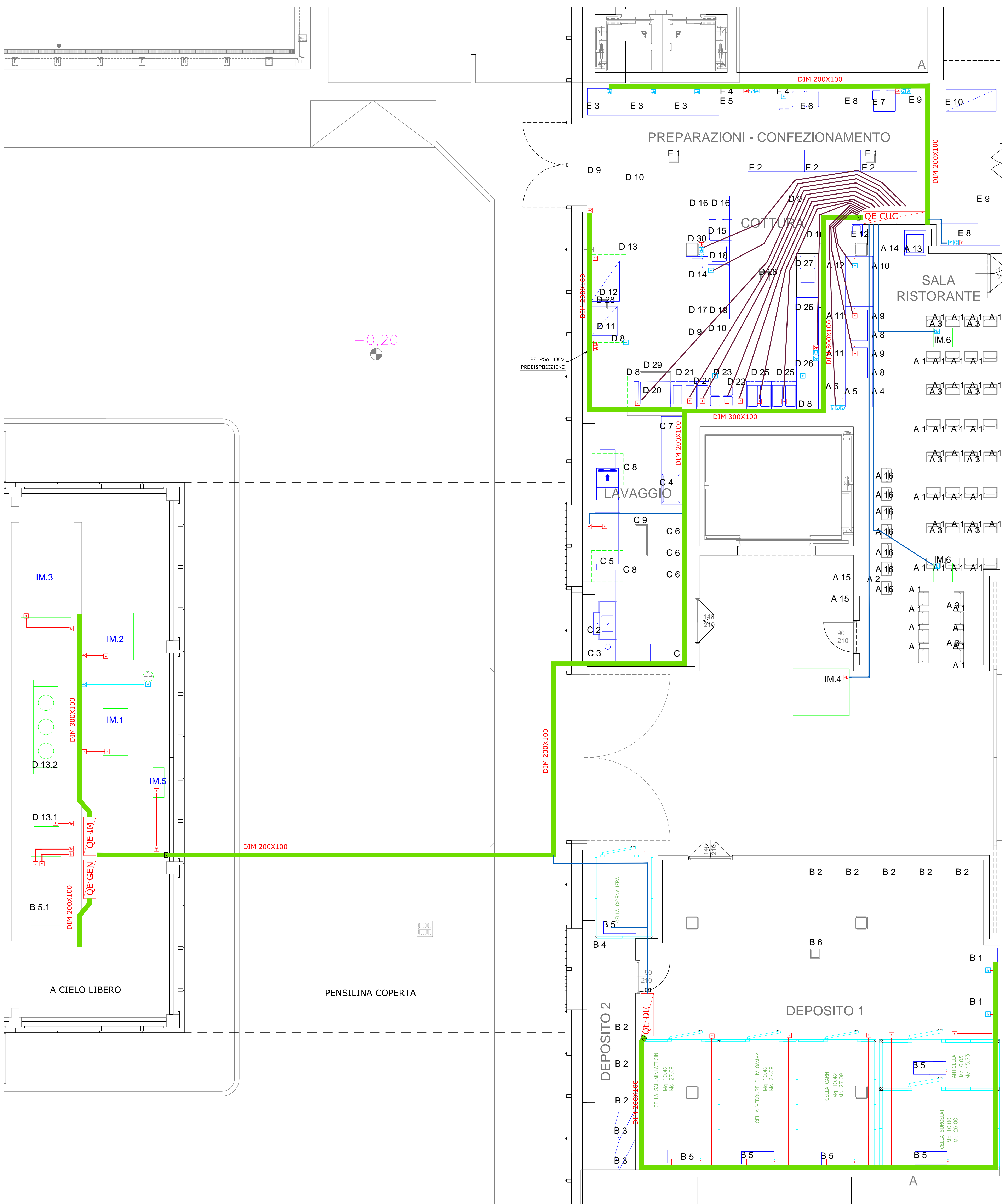
PLANIMETRIA IMPIANTO FM - SCALA 1:50
